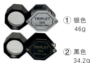
KYG0297 10倍六角形放大镜 Loupe 10X \times 20.5mm
