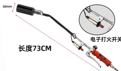
KYG1486 焊枪 Torch 长度73cm 接内径50mm 外径8mm皮管
