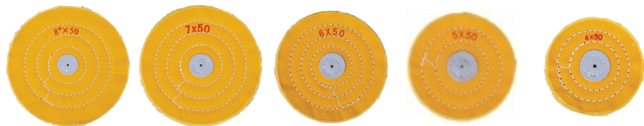
KYG1239 黄布轮 Yellow Buffs No:8"×50 KYG1240 黄布轮 Yellow Buffs No:7"×50 KYG1241 黄布轮 Yellow Buffs No:6"×50 KYG1242 黄布轮 Yellow Buffs No:5"×50 KYG1243 黄布轮 Yellow Buffs No:4"×50
