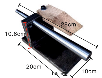
KYG1090 便携式执模台 Portable Mold Holder
