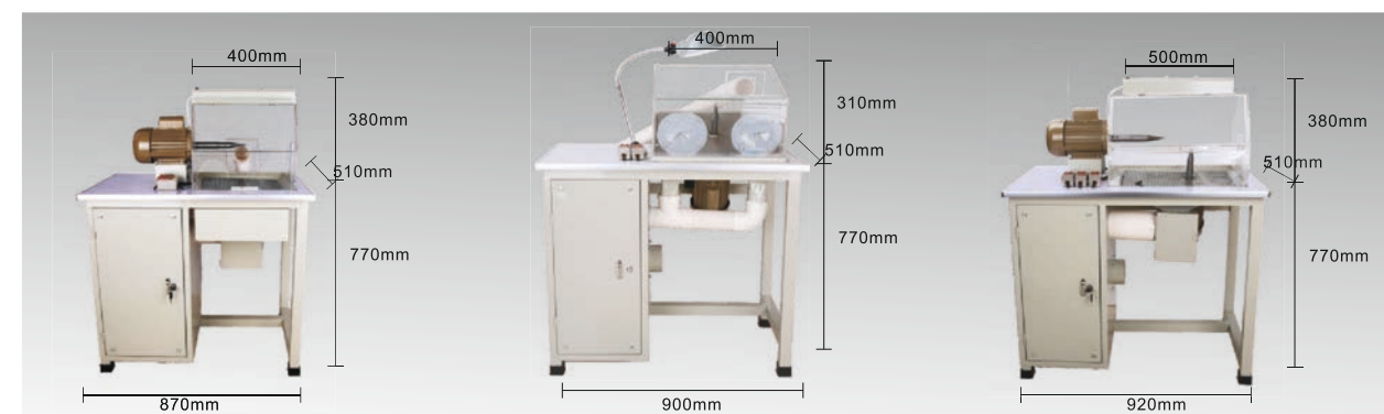
KYG0768 单位吸尘打磨机 Polishing Machine 打磨功率Power: 550W 吸尘功率Polishing power: 550W 电压Voltage: 220V 重量Weight: 55kg
