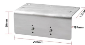
KYG0126 台面定位铁 Optional Mounting Adapter 重量Weight:1.5kg
