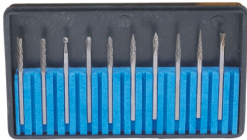
KYG1215 钨钢锉(套装) Tungsten Carbide Rotary Files 锉头Size \phi : 2.35mm 柄径 \phi : 2.35mm 长度L: 50mm
