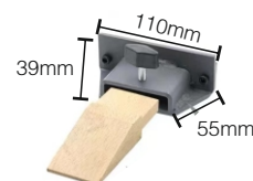
KYG0127 台塞固定铁 Bench Pin Kit 重量Weight:1.95kg
