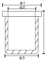
KYG1510 石墨坩(五星材质) Graphite Crucible
